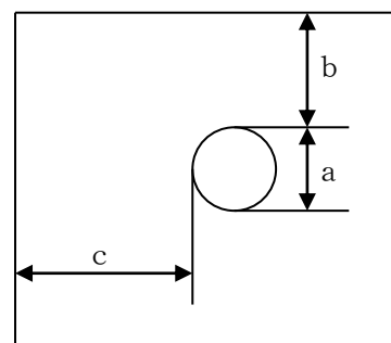
令8-1号区画の端部と開口部の離隔距離
