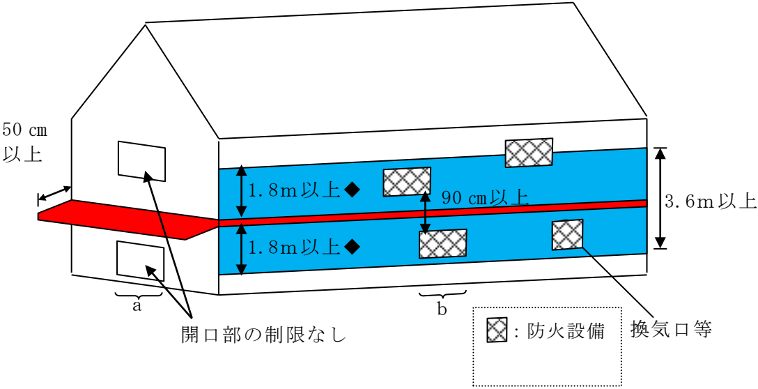
(立面図)
