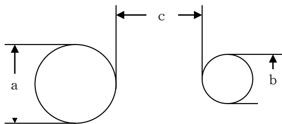
開口部相互の離隔距離
