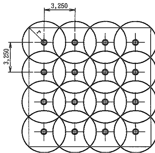
第4-5図 格子配置 r 2.3 の場合
