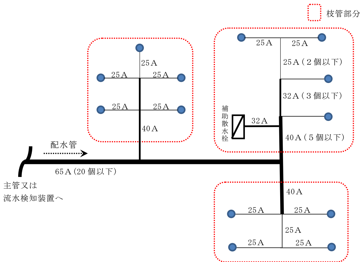
第 4－4 図 配置の設置例：標準型ヘッドの場合
