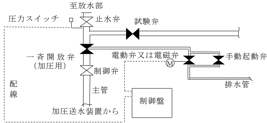
第4-17図（加圧方式の一斉開放弁等の廻りの配管図例）
