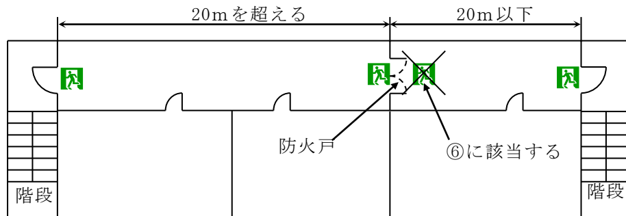
第17-23図 避難口誘導灯の設置緩和例
