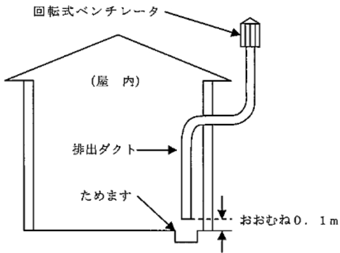
第 15-10 図 強制排出設備の例
