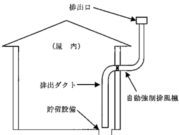
第15-8図 自動強制排出設備の例
