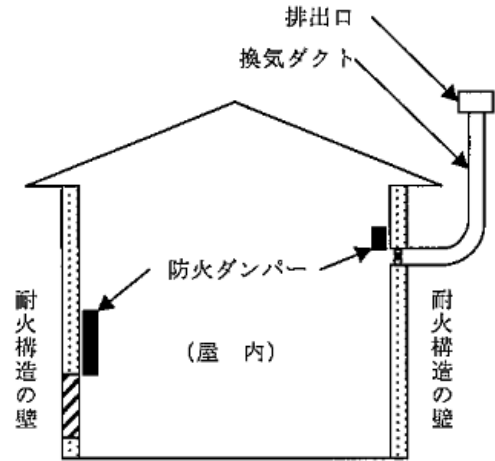
第15-6図 防火ダンパーの設置例
