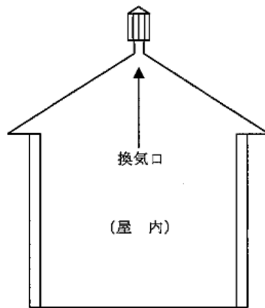
第 15-2 図 強制換気設備の例
