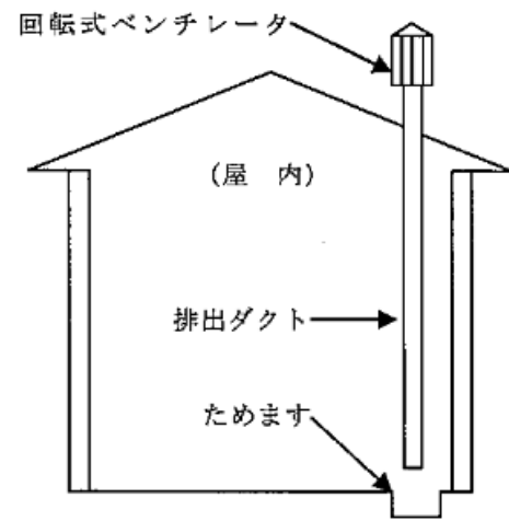
第 15-11 図 強制排出設備の例
