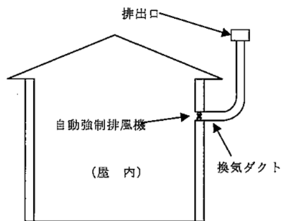
第 15-4 図 自動強制換気設備の例
