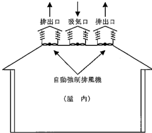
第15-5図 自動強制換気設備の例
