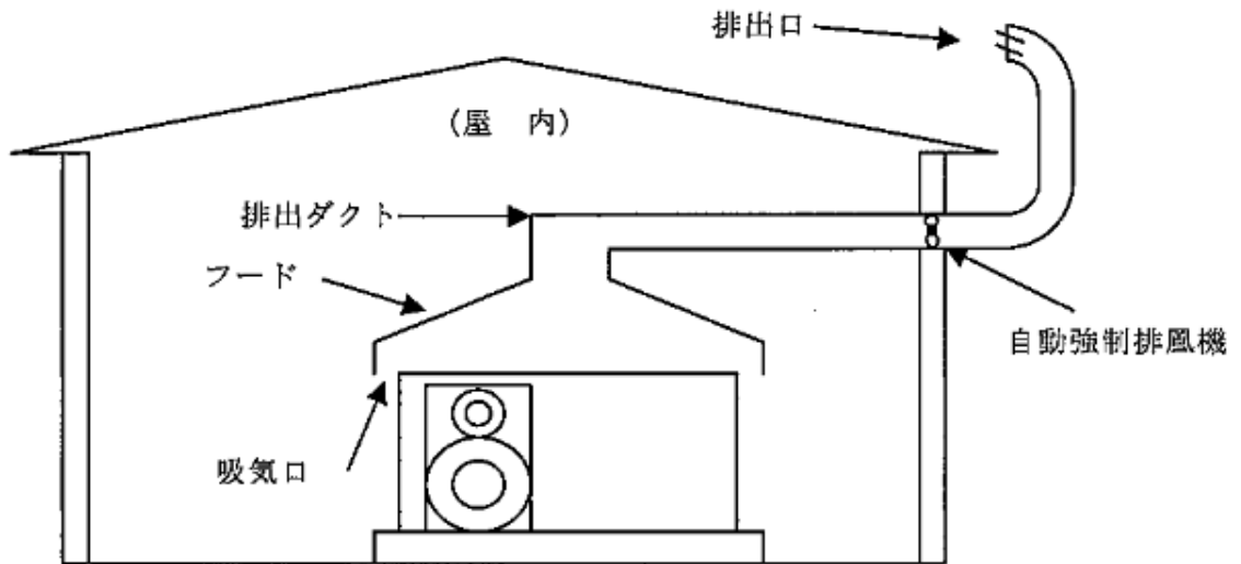
第15-7図 自動強制排出設備の例
