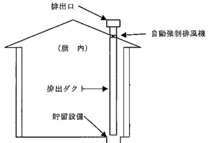
第15-9図 自動強制排出設備の例
