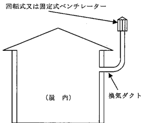
第 15-3 図 強制換気設備の例
