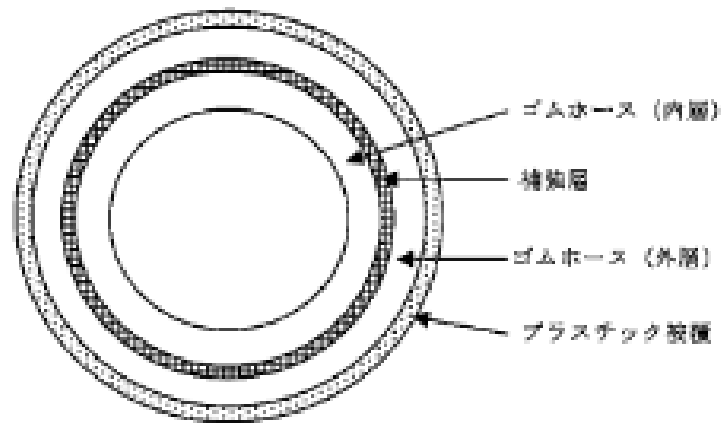
第 12-21 図 プラスチックで被覆された給油ホース等の構造 (断面)
