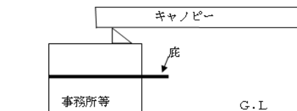
第12-1図 上屋面積の算定例
