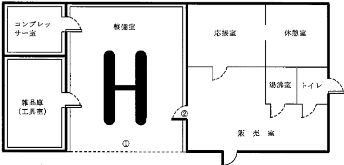
第12-14図 内部構造例 耐火構造又は不燃構造の部分を示す。
