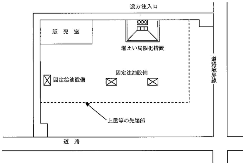
第 12-37 図 固定給油設備等設置例
