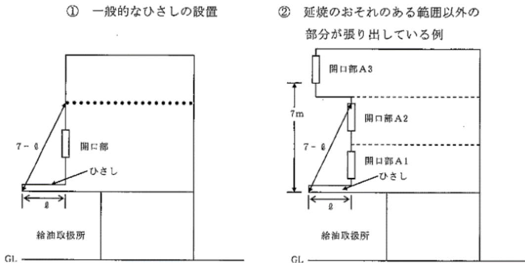
第 12-39 図 延焼防止上有効な屋根又はひさしの設置例
