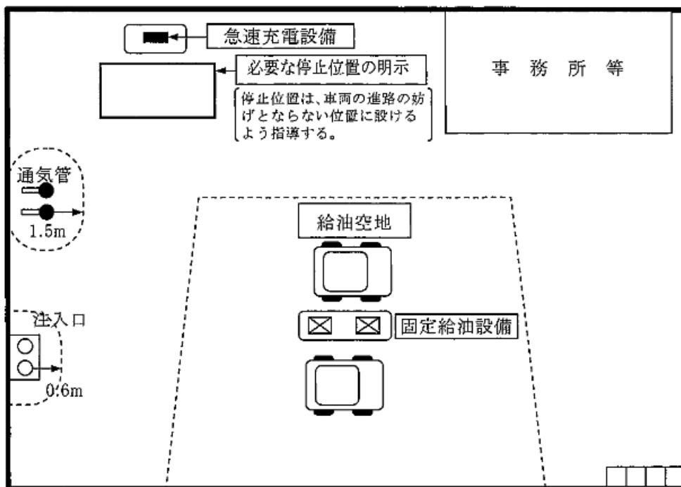
第 12-64 図 給油取扱所における急速充電設備の設置例
