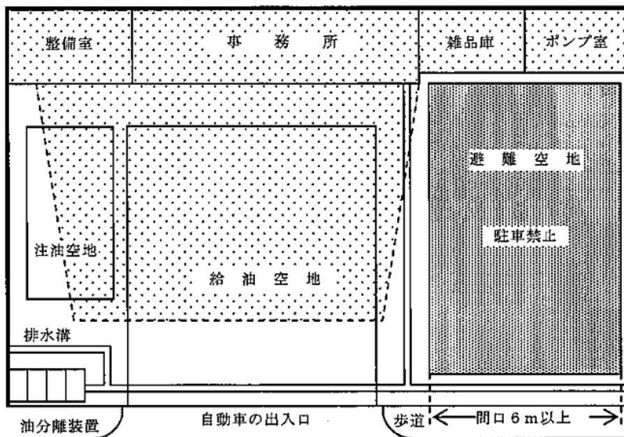
第12-29図 避難空地
