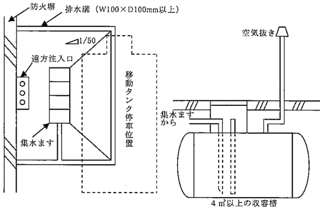
第12-38図 漏えい局限化措置の例
