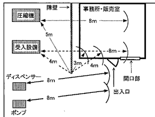
第 12-51 図 建築物の出入口、開口部による迂回距離によって 8m 以上となる例
