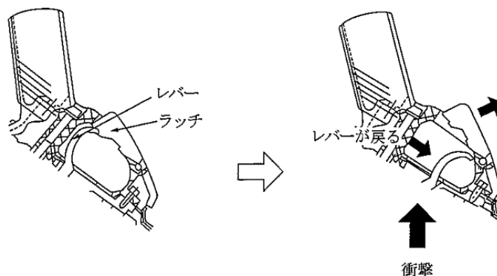
第 12-58 図 脱落時停止制御装置の作動例
