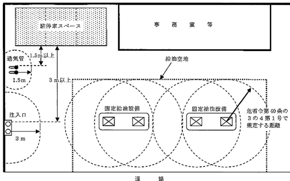
第12-25図 駐車スペースの例
