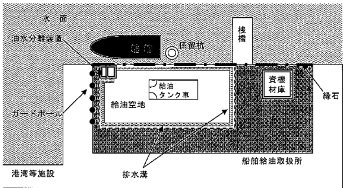
第 12-42 図 船舶給油取扱所の設置例
