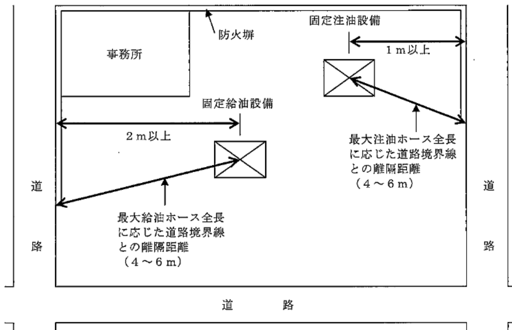
第 12-18 図 固定給油設備等の位置
