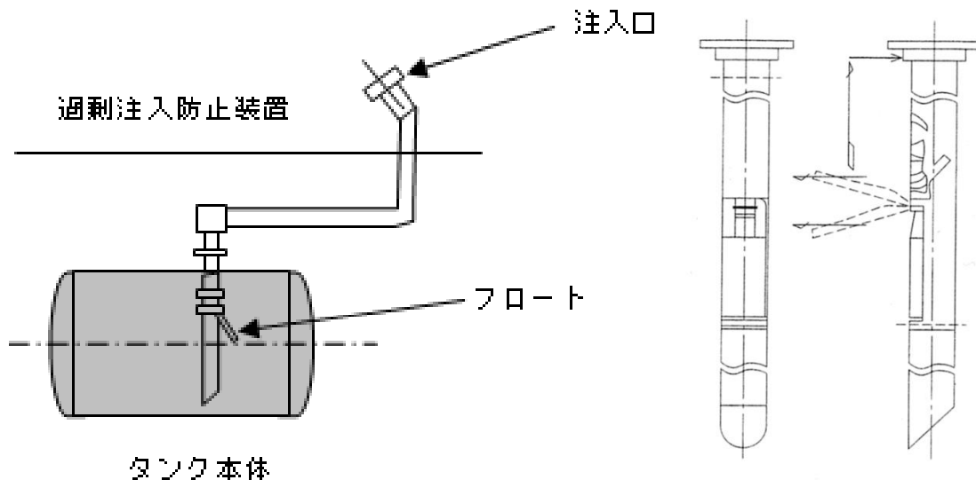
第12-30図 過剰注入防止装置（フロート式）
