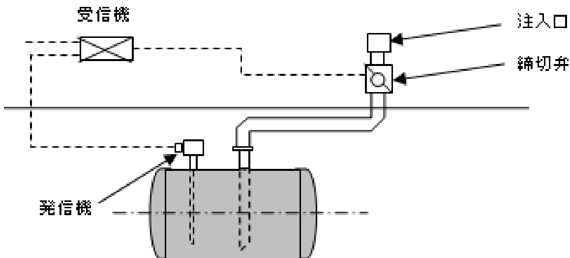
第12-31図 過剰注入防止装置（締切弁方式）
