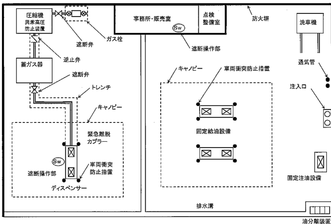
第 12-49-2 図 屋外給油取扱所に圧縮天然ガス充てん設備を併設した例
