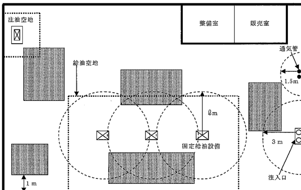
ℓ：危省令第25条の5第2項第2号イに規定する距離 第12-27図 作業場所等（網掛け部分）として認められない設置例
