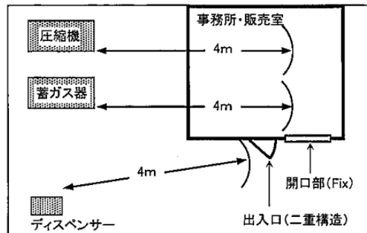
第12-46図 4m未満に建築物の出入口、開口部がある例
