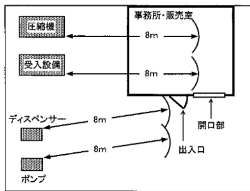
第 12-50 図 8m 未満に建築物の出入口、開口部がある例
