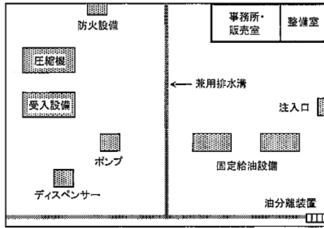
第 1 2 - 5 3 図 危険物用と防火設備用の兼用排水溝の設置例
