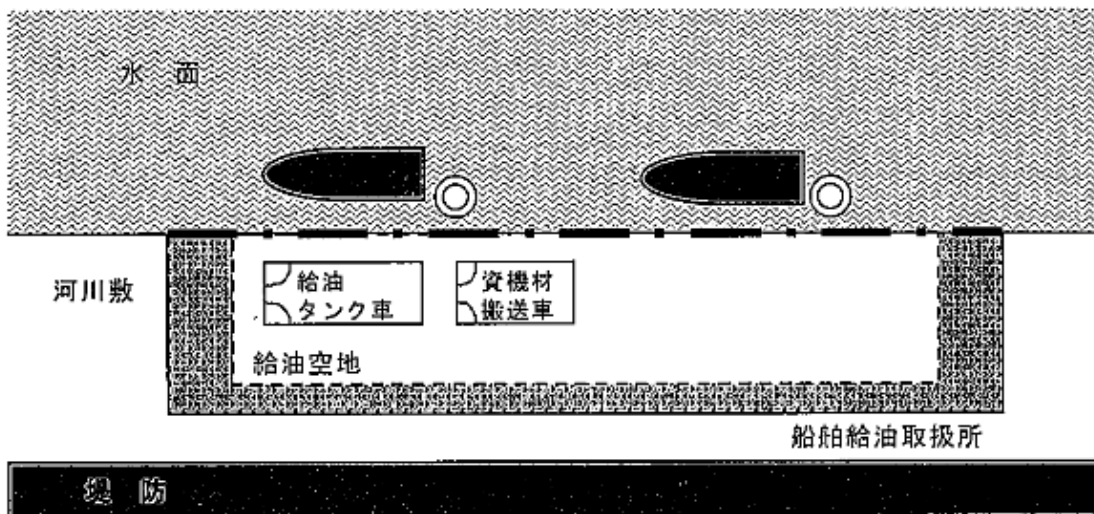
第 12-44 図 給油時に流出防止設備等の資機材を搬送する場合の設置例
