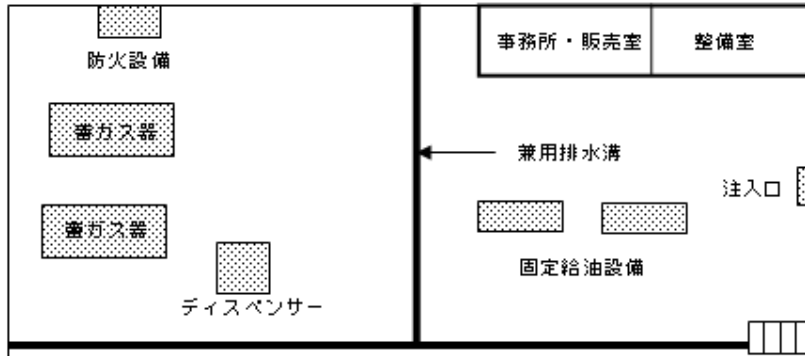
第 12-49 図 危険物と圧縮天然ガススタンド用の兼用排水溝の設置例
