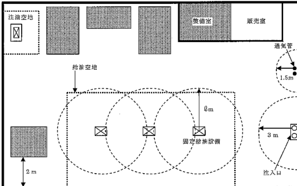
ℓ：危省令第25条の5第2項第2号イに規定する距離 第12-26図 作業場所等（網掛け部分）として認められる設置例
