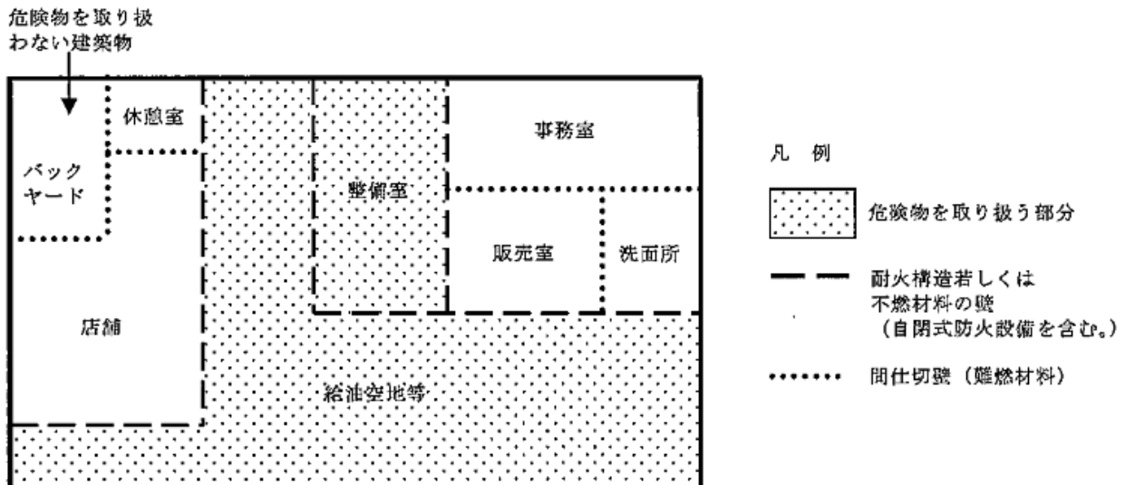
第 12-11 図 不燃材料以外の建築材料で造ることのできる間仕切り壁の例
