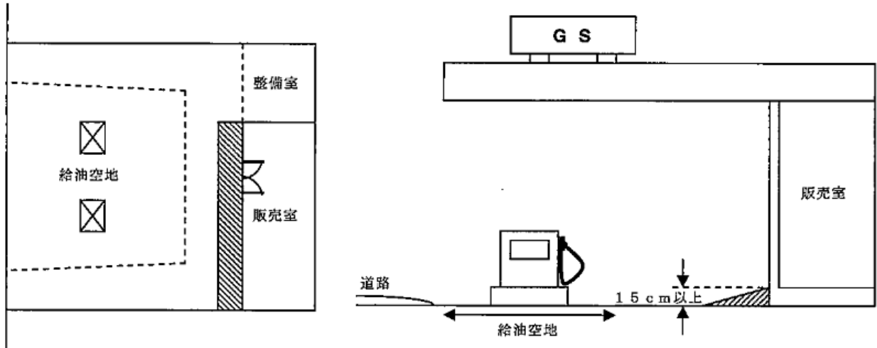
第12-15図 コンクリート製スロープ設置例
