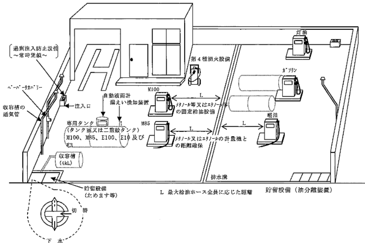
第12-57図 ガソリン等とメタノール等又はエタノール等を取り扱う給油取扱所の設置例
