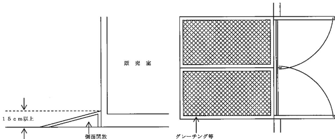
第12-16図 可燃性蒸気滞留防止構造例
