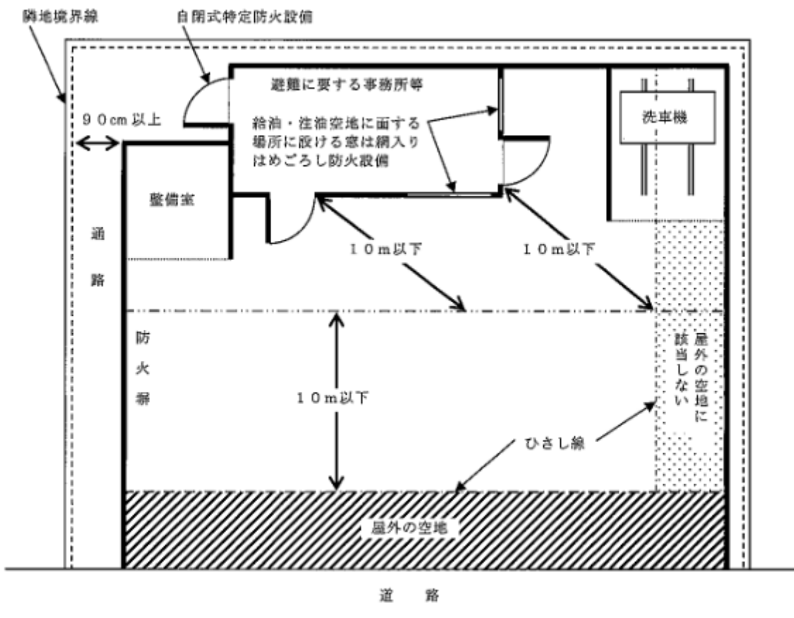
第12-32図 避難通路の確保例
