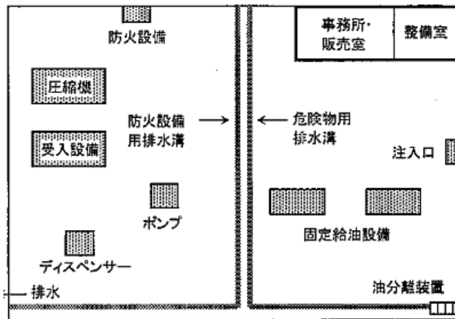
第 1 2 - 5 3 - 1 図 危険物用と防火設備用の排水溝を別々に設置した例
