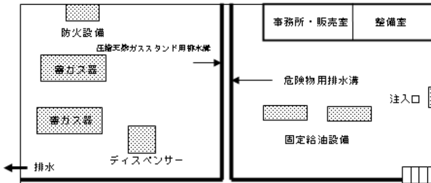
第 12-49-1 図 危険物用と圧縮天然ガススタンド用の排水溝を別々に設置した例
