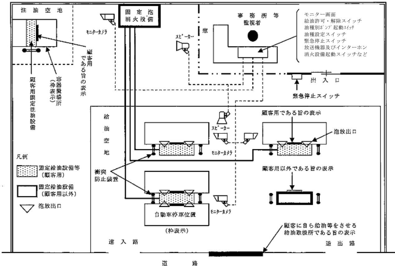
第 12-63 図 セルフ給油取扱所の設置例
