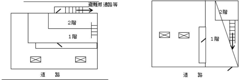
第 12-11 図 敷地外へ直接避難できる構造例
