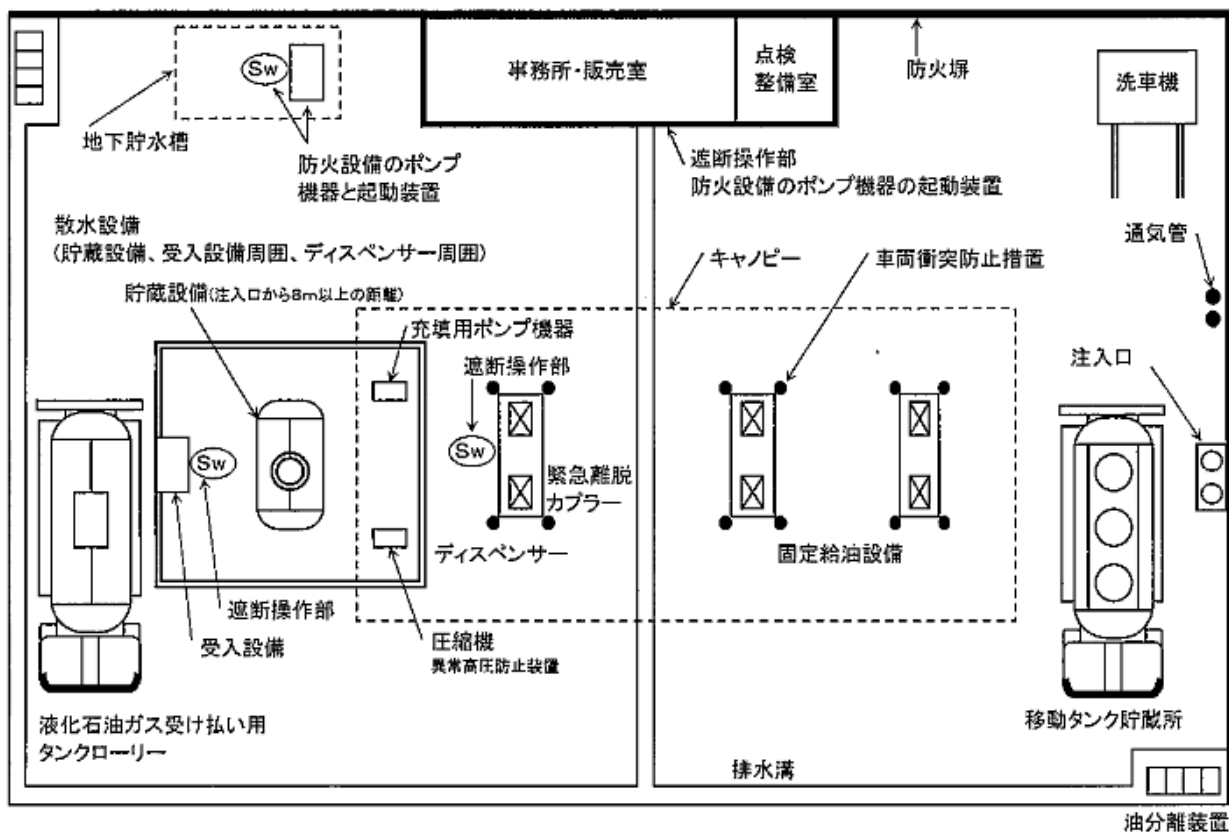
第 12-53-2 図 屋外給油取扱所に液化石油ガススタンドを併設した例
