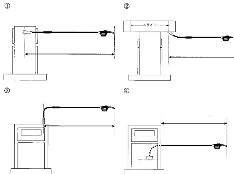
第12-22図 給油ホース等の全長
