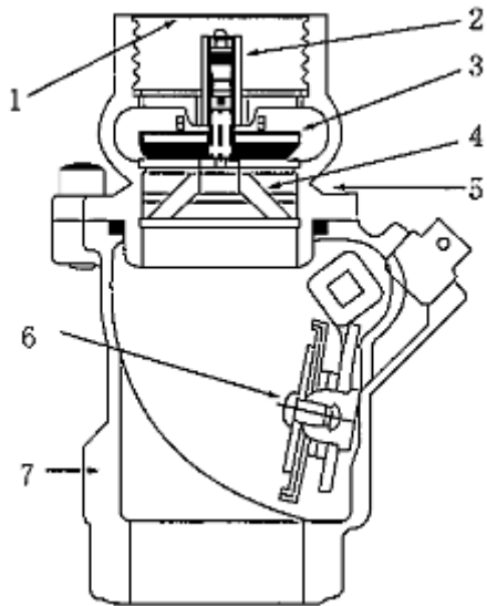
第 12-60 図 立ち上がり配管遮断弁の構造例
