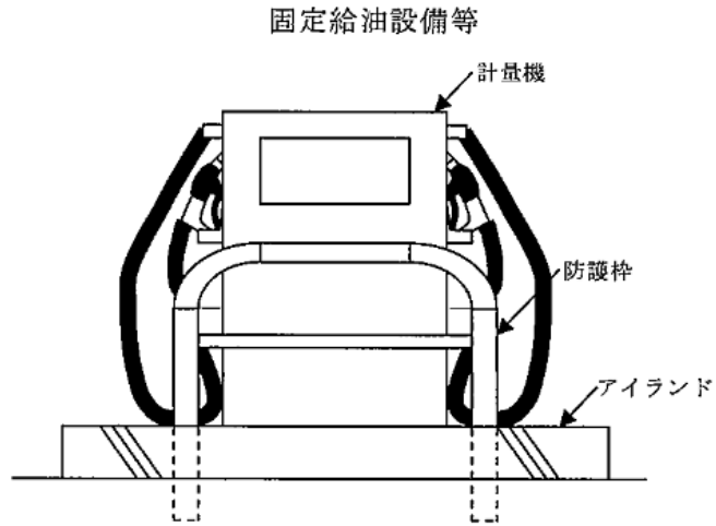
第 12-33 図 衝突防止措置の例
