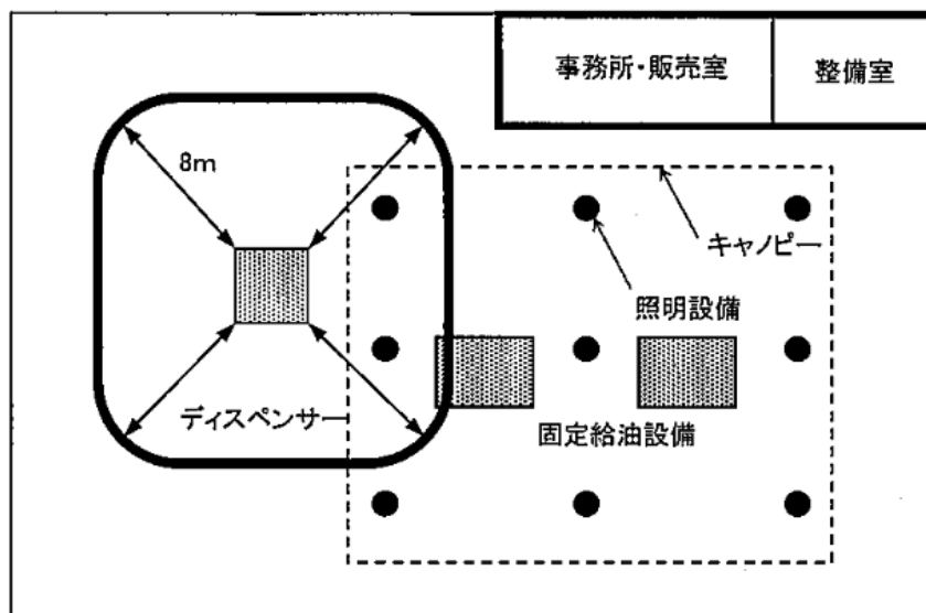
第12-52図 電気設備に耐圧防爆措置が必要な範囲 (ディスペンサー外部から8mの範囲内の電気設備が全て対象)
