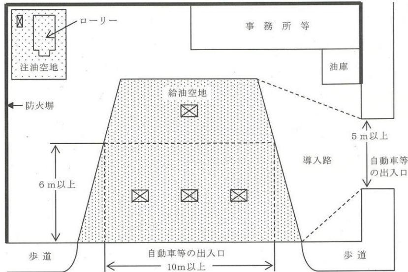
第12-7図 給油空地及び注油空地の例
