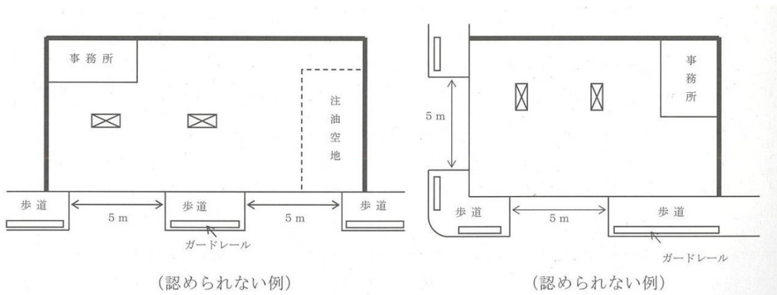
第12-3図 自動車の出入口
