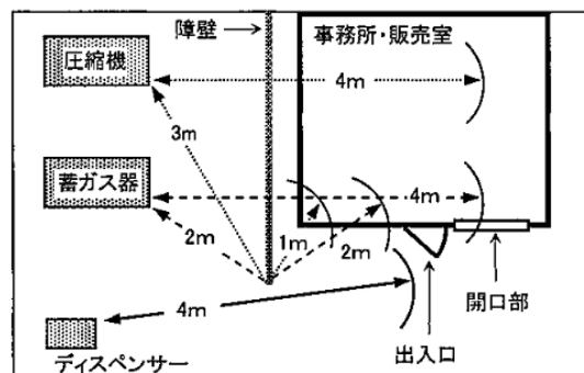
第12-46-1図 建築物の出入口、開口部が障壁による迂回距離によって4m以上となる例
