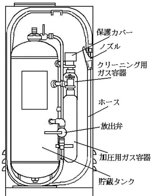
移動式粉末消火設備 (加圧式)
